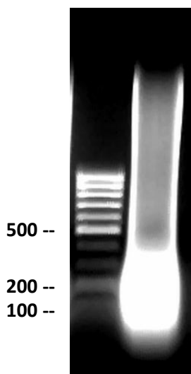
Elektroforeogram
